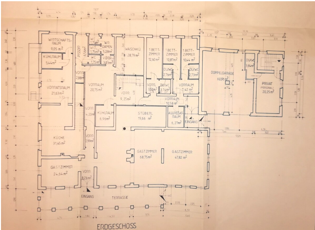
Plan Erdgeschoss
